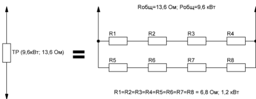
Схема эквивалентного блока резисторов без изменения тормозного момента, но имеющим небольшой запас по мощности
